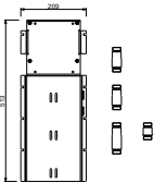
ESEMPI DI COMBINAZIONI - 3 USCITE
