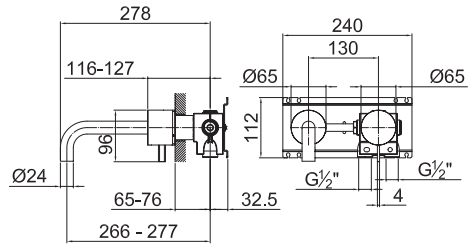
ART. A613A Parte incasso / Built-in pieces / Partier à encastrer / Eingebaute Stücke / Pedazos incorporados / Встроенная часть
