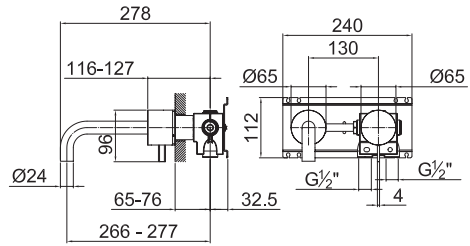
ART. A613B Parte esterna / External pieces / Parties externes / Up-Teil / Parte externa / Наружная часть
