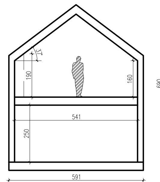
SCHEMAT PRZEKROJU/ SECTION SCHEME
