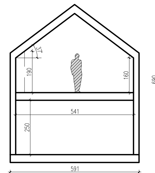
SCHEMAT PRZEKROJU/ SECTION SCHEME
