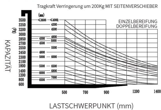
DIAGRAMM DER NENNKAPAZITÄTEN UND LASTSCHWERPUNKTE
