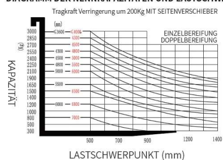
DIAGRAMM DER NENNKAPAZITÄTEN UND LASTSCHWERPUNKTE
