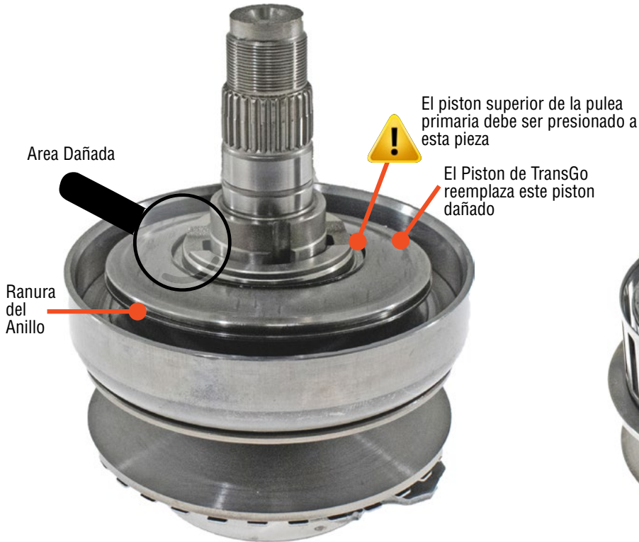
Ensamble de la pulea primaria
