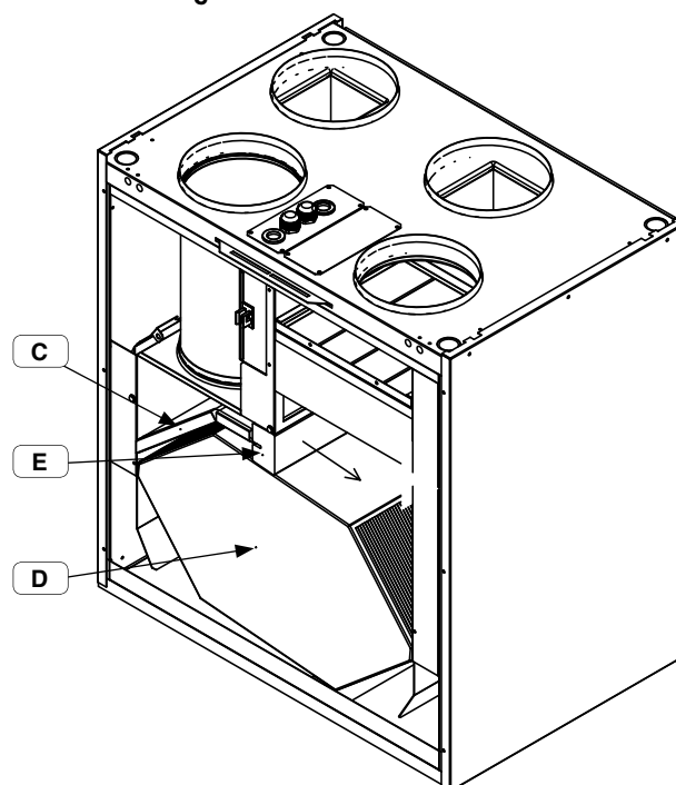
Värmeåtervinningselement
