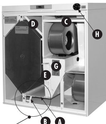
Vaihtopelti kesäasennossa
