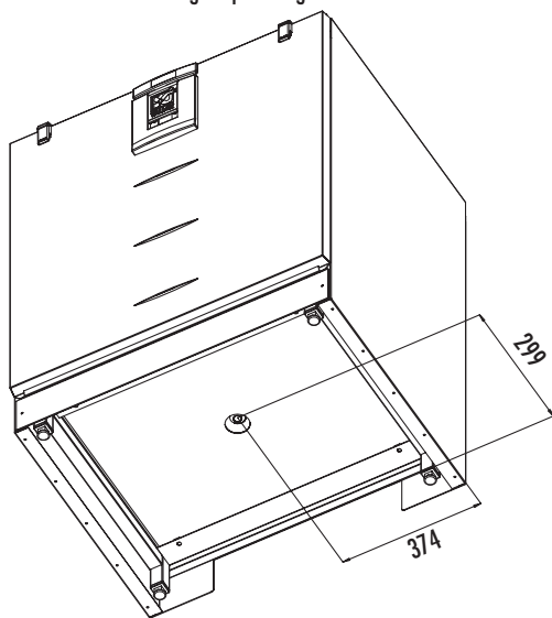
Kondensvattenanslutningens placering
