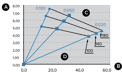
Vallox 245 MV жидкостный радиатор t_{\text{air}}=15^\circ\text{C} , t_{\text{fl}}=85^\circ\text{C}
