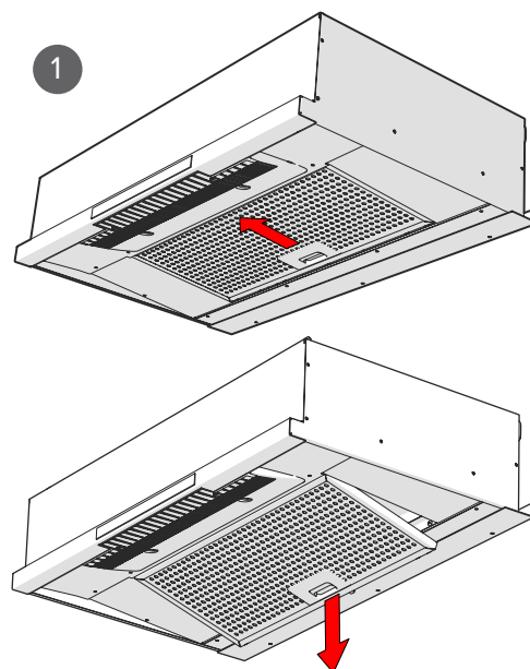
Filtro išėmimas
