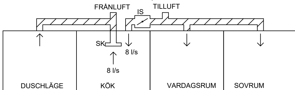
NORMAL KÖKSVENTILATION VIA SPISKÅPAN, SKÅPANS SPJÄLL STÄNGT
