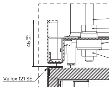
Huoneen katto saa olla 40 mm alempana kuin kattoasennuslevyn valkoisen peitelistan yläreuna
