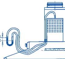
Tehostusilmavirran mittaus
