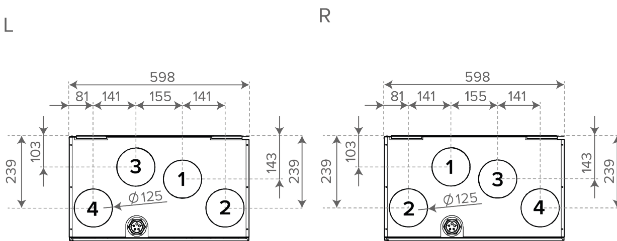
Kuva 6. Kanavalähdöt, L-malli ja R-malli
