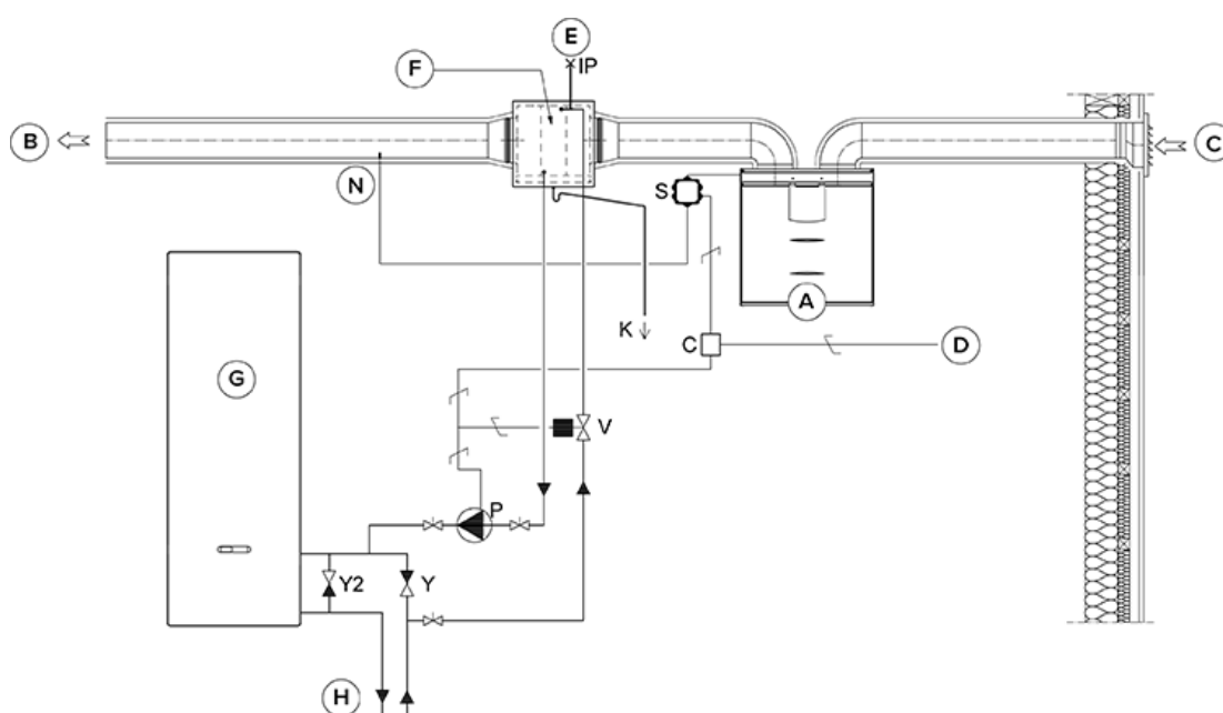
Kuva 4. Kanavapatterin toimintakaavio tuloilmakanavassa
