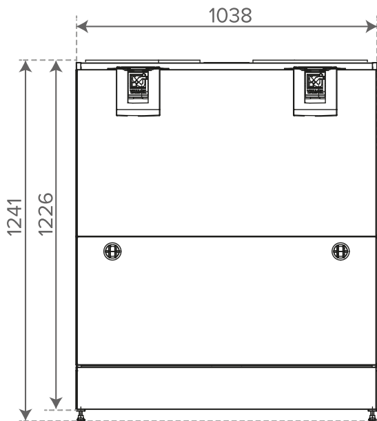
Kuva 9. Kanavalähdöt
