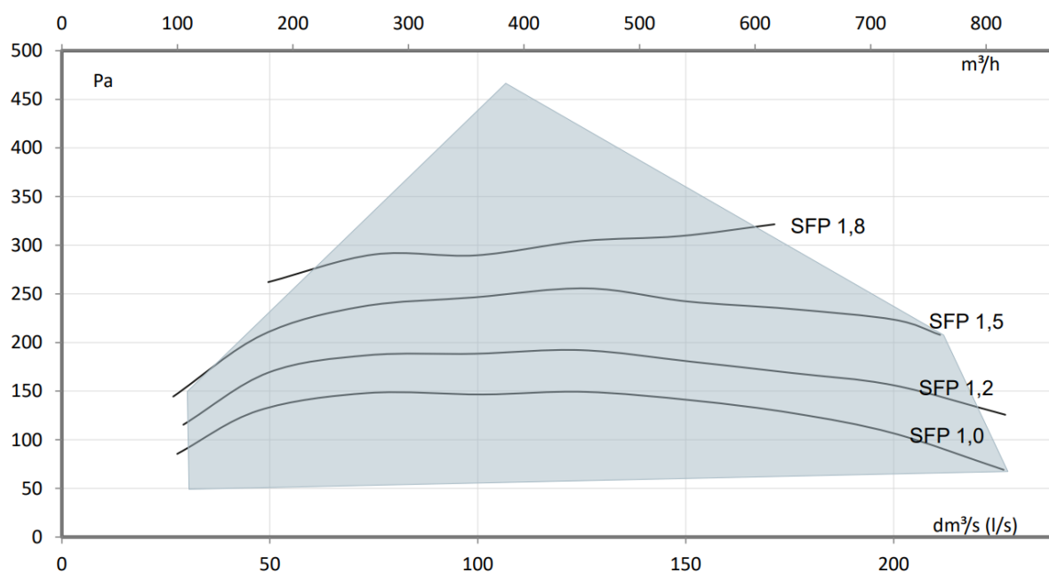
Kuva 2. Puhaltimen tulo- ja poistoilmamäärät, entalpiakenno
