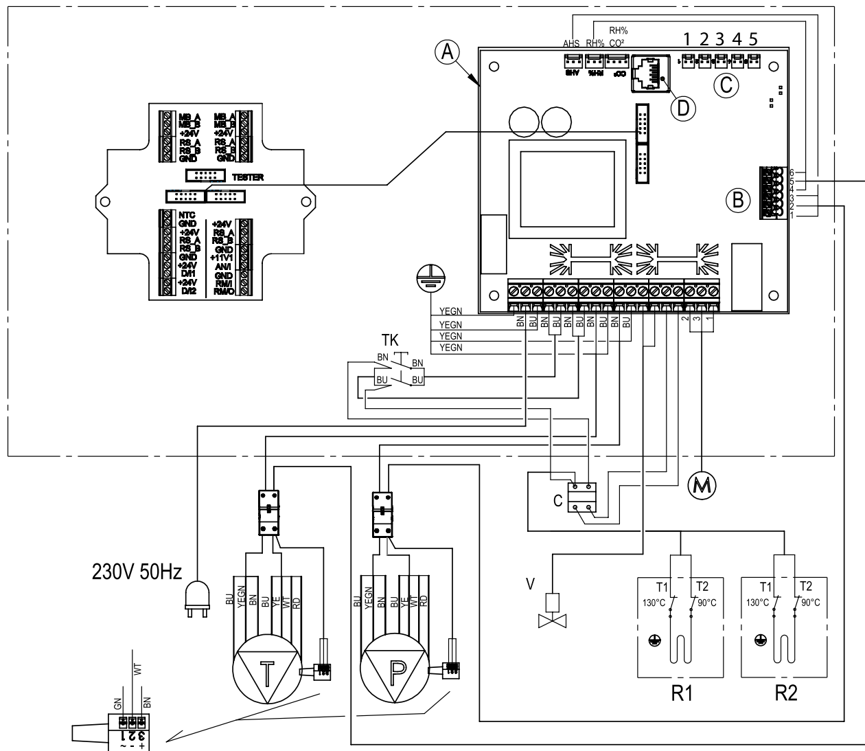
Kuva 5. Sisäinen sähkökytkentä MyVallox 245 CFi VKL
