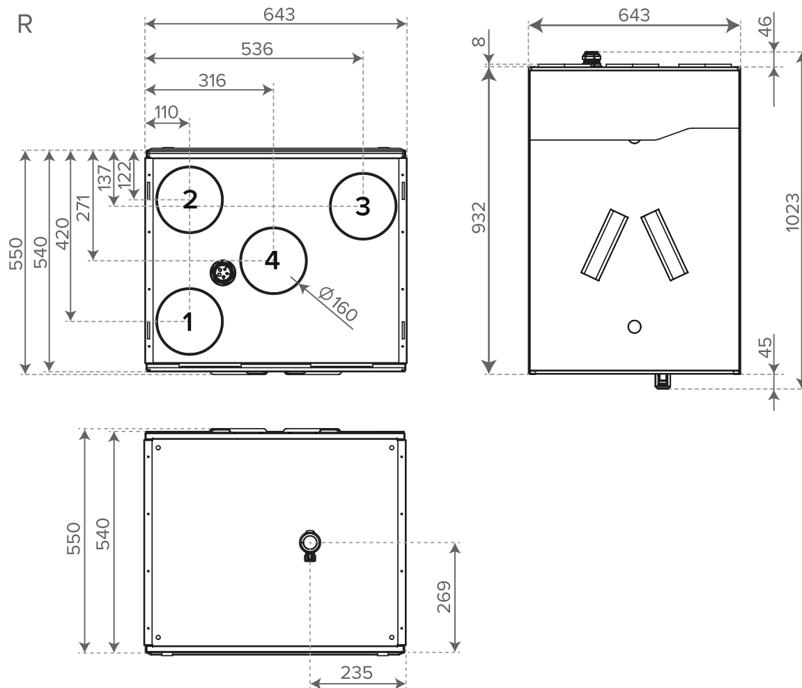
Figur 7. Mått och kanalstosar MyVallox 119 CFI R
