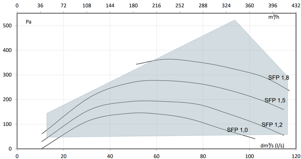
Figur 4. Fläktarnas tillufts- och frånluftsmängder, entalpivärmexlare
