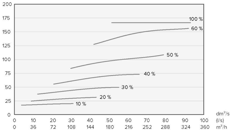
Figure 2. Fan input power
