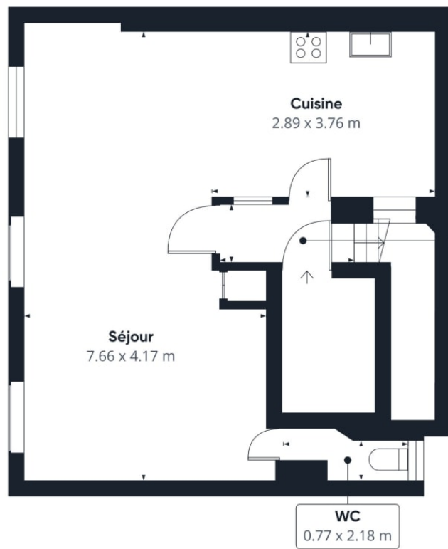
Niveau 0
