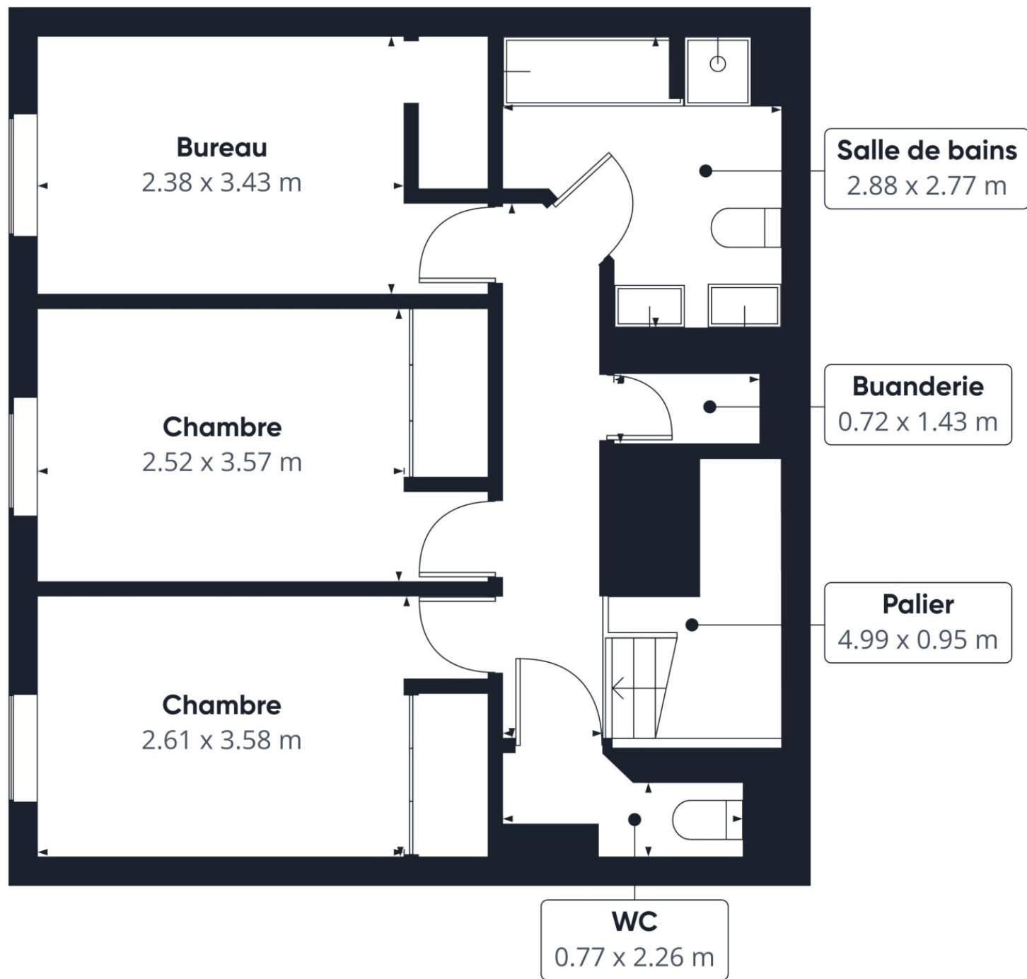
Niveau 1
