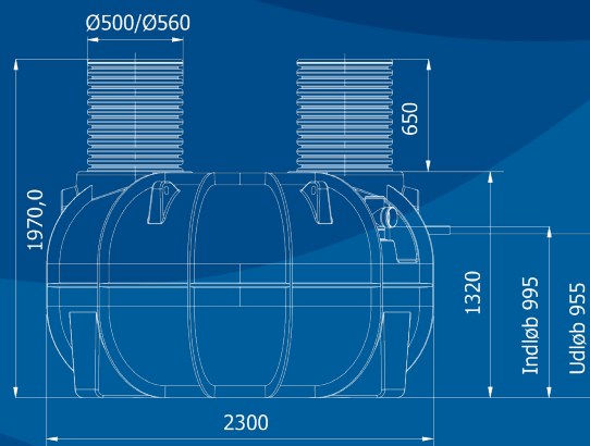
5 PE Bundfældningstank, 223193126-128
