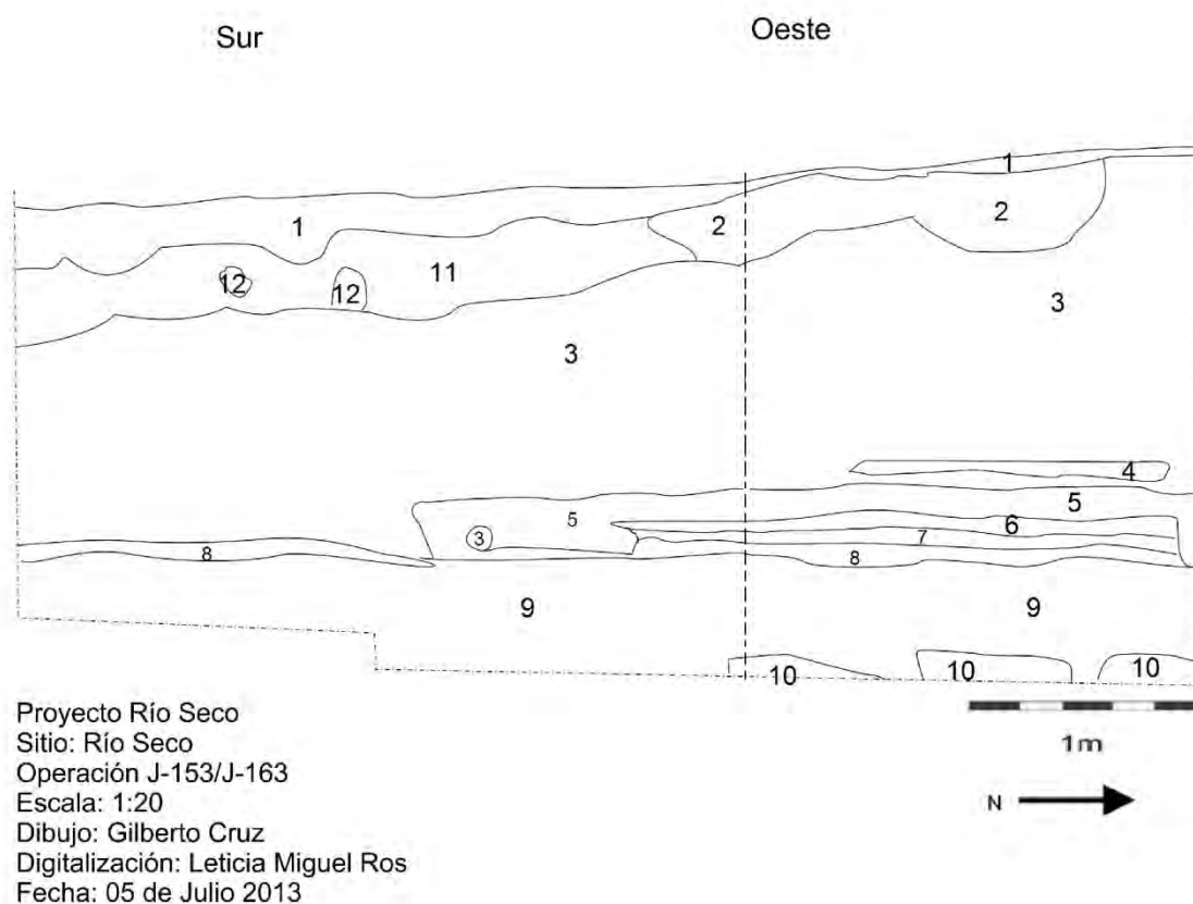
Figura A1.18. Dibujo de los perfiles Sur y Oeste de la Operación J-153/J-163 (Dibujo por G. Cruz y digitalización por L. Miguel Ros).
