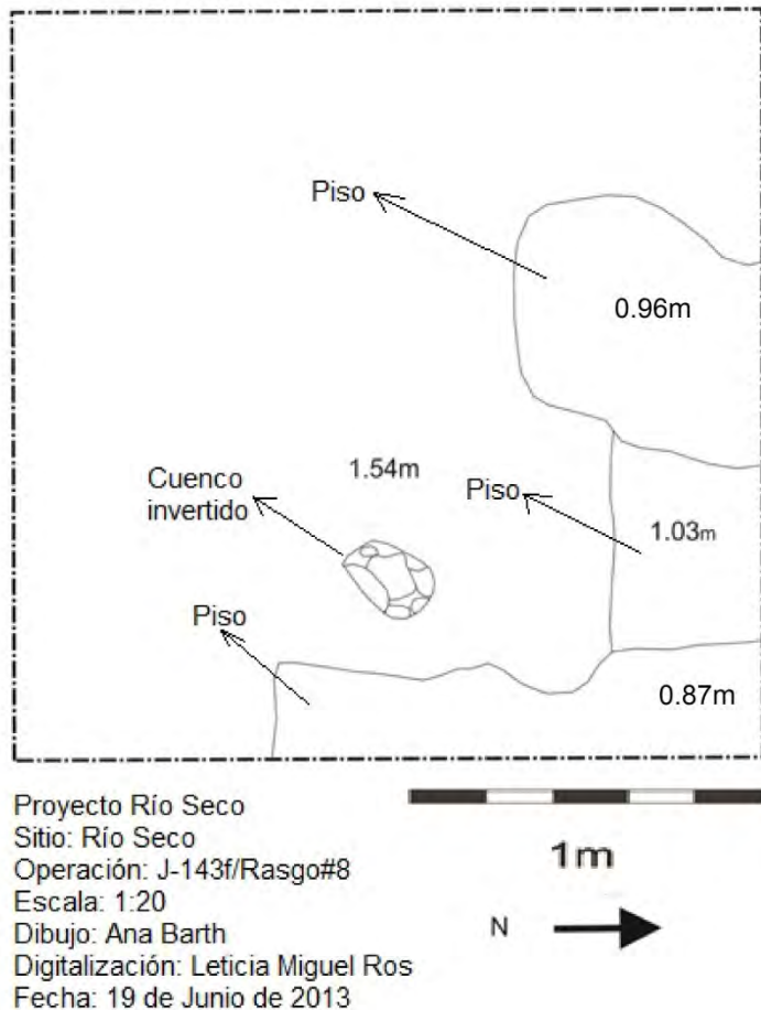
Figura A1.8. Dibujo de planta del Rasgo #8 en Operación J-143f (Dibujo por A. Barth y digitalización por L. Miguel Ros).
