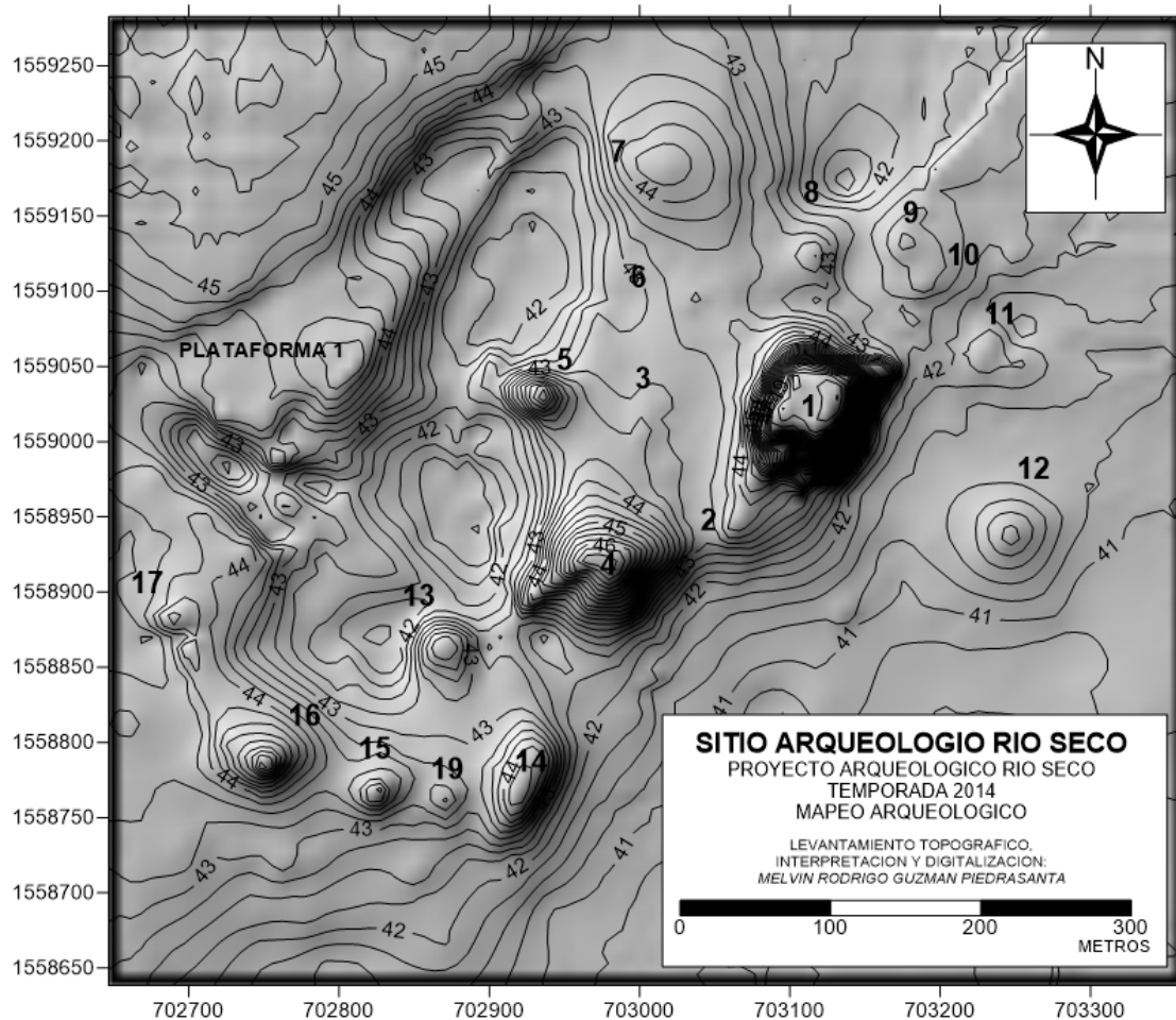
Figura 7.1. Plano de curvas de nivel en donde se aprecian los volúmenes que representan los montículos del sitio. Los números grandes en negrilla corresponden al número de montículo (Mapa por R. Guzmán) (Guzmán en este informe).
