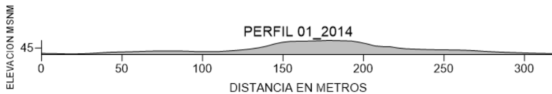
Figura 2.7. Perfil 01 del mapa (Elaborado por R. Guzmán).
