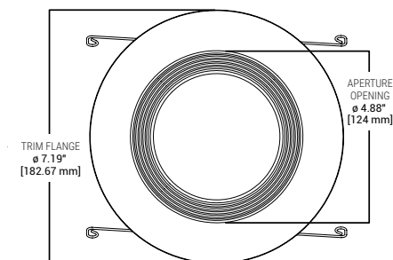
LT56 - 750 Lumen
