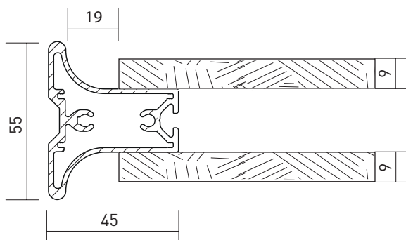
Flächenfüllungen aufliegend frame panels both sides
