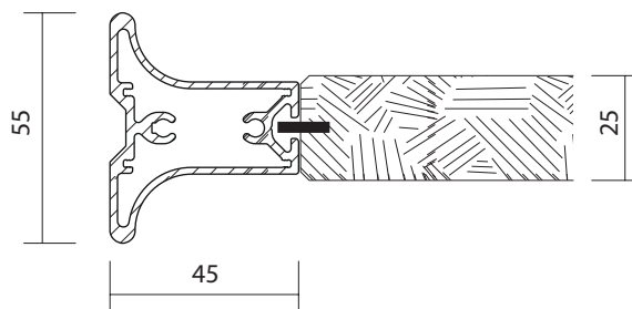
Flächenfüllungen innenliegend frame panels in frame
