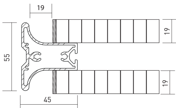
Flächenfüllungen aufliegend frame panels both sides
