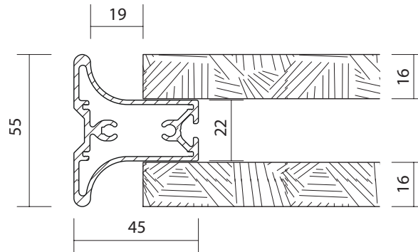
Flächenfüllungen aufliegend frame panels both sides
