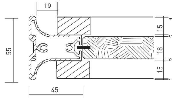
Flächenfüllungen aufliegend frame panels both sides
