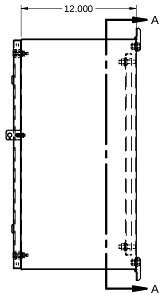
SIDE / CÔTÉ
