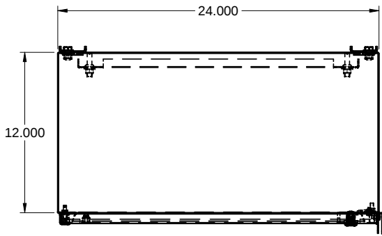
TOP / DESSUS
