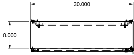
TOP / DESSUS
