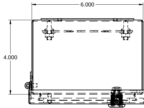
TOP / DESSUS
