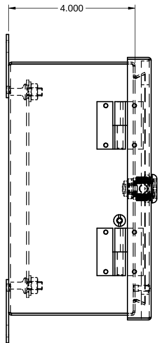
SIDE / CÔTÉ
