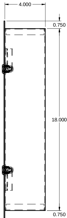
SIDE / CÔTÉ
