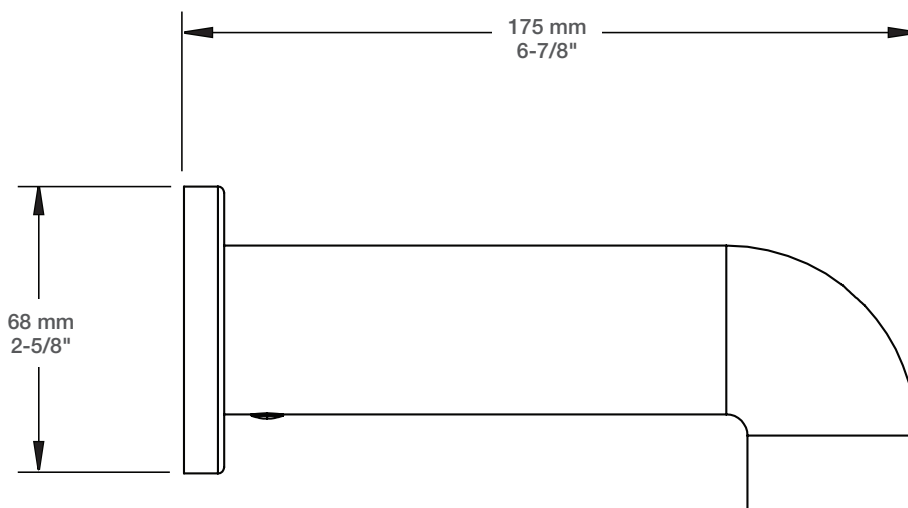
Installation « slip-fit » Slip-fit installation
