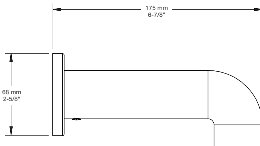
Installation « slip-fit » Slip-fit installation
