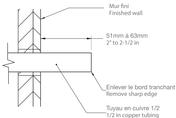
Installation « slip-fit » Slip-fit installation
