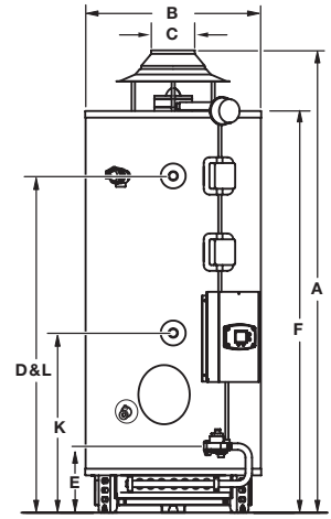
D-75T-300 D-65T-(370, 399) D-80T-(425, 505)
