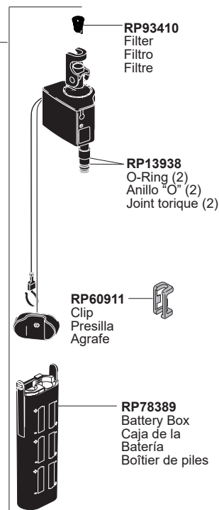
EP92546 Solenoid Assembly Ensamble de Solenoïde Électrovanne
