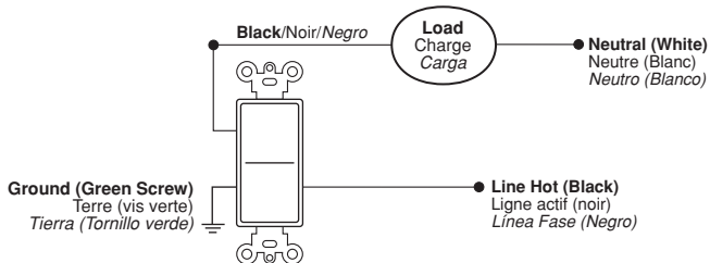
Wiring Diagram/Schema de câblage/Diagrama de Cableado
