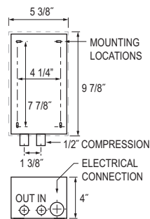
Single Module
