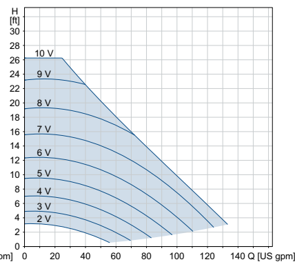
0-10 volts*
