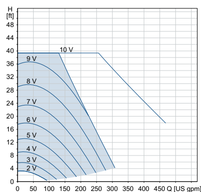
0-10 volts*
