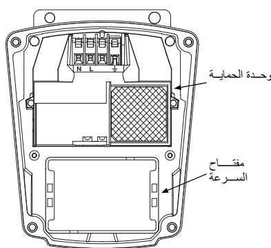
شكل 3 صندوق التوصيلات UPS 115 × 1 فولت و 230 فولت
