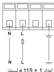
إمداد 115 × 1 فولت
