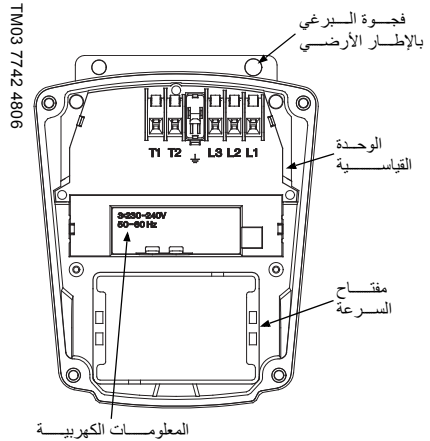
شكل 21 صندوق التوصيل
