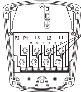
شكل 8 صندوق توصيل UPS 3 x 460 فولت و 575 فولت
