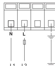
إمداد 230 × 1 فولت
