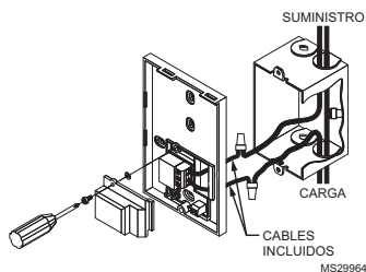
Fig. 2. Trazado de los cables hacia el termostato.
