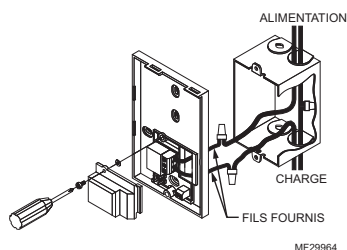
Fig. 2. Acheminement des fils vers le thermostat.
