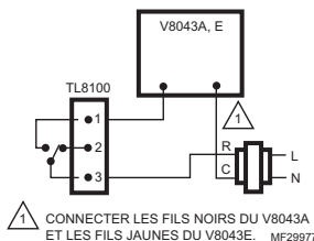
Fig. 7. Schéma de câblage d'une vanne à deux fils de 24 V c.a. (V8043A,E ou équivalente).
