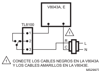
Fig. 7. Diagrama de cableado de una válvula de 2 cables, de 24 V CA (V8043A, E o equivalente).
