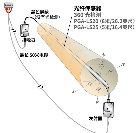
PGA-LS20：有效长度为8米 PGA-LS25：有效长度为5米 PGA-LS30：有效长度为18米
