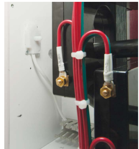
点传感器正确安装示例。
