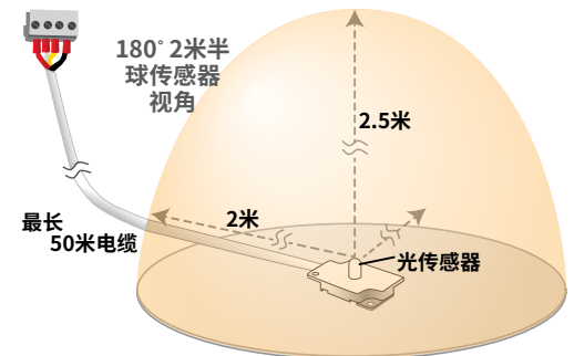
PGA-LS10： 3 kA电弧故障的检测范围
