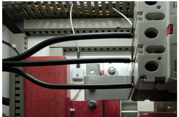
光纤传感器正确安装示例。
