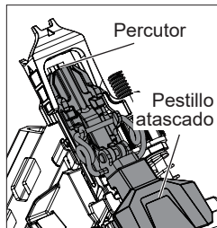
PESTILLO DE ATASCO CERRADO
