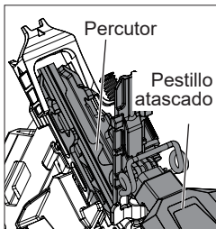
ATASCO DE PESTILLO ABIERTO
