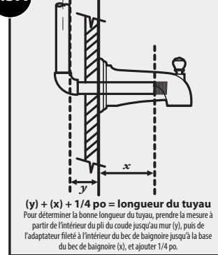
4.3A Installation du bec de baignoire
