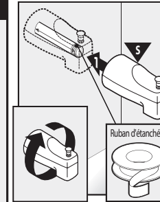
4.3A Installation du bec de baignoire
