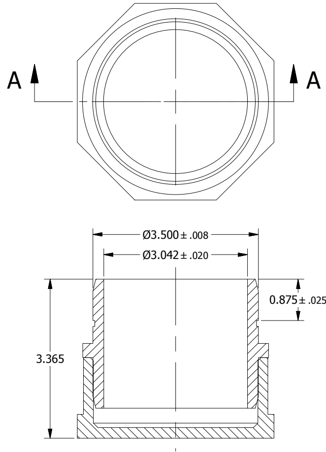
SECTION A-A
