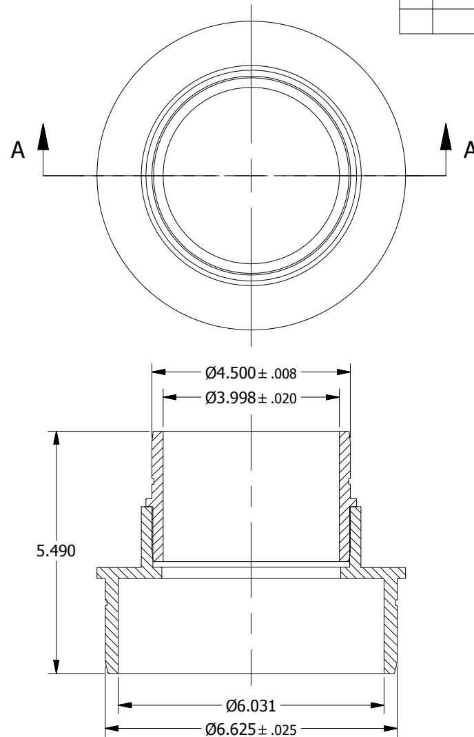
SECTION A-A
