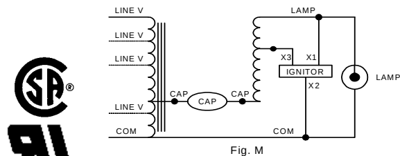
Wiring Diagram:
