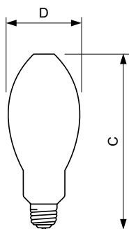
MHC 70W/930 E26 BD17 CO U ELITE
