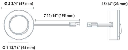
1 Wire
