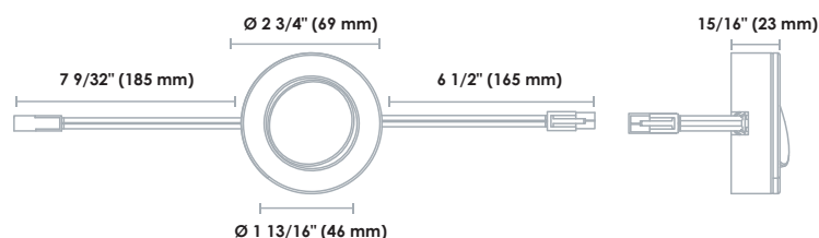
2 Wires
