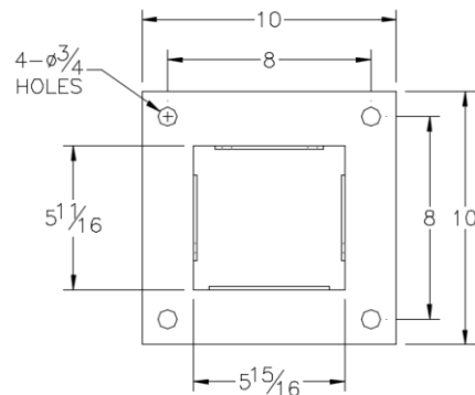
EXTERNAL BASEPLATE (Add Suffix -EB to Part #)
