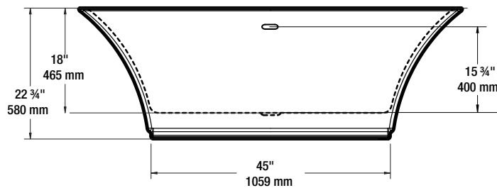
FRONT VIEW VUE DE FACE
