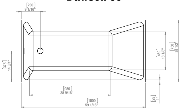
TOP VIEW VUE DE DESSUS
