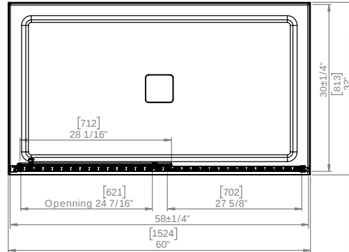
TOP VIEW VUE DU HAUT
