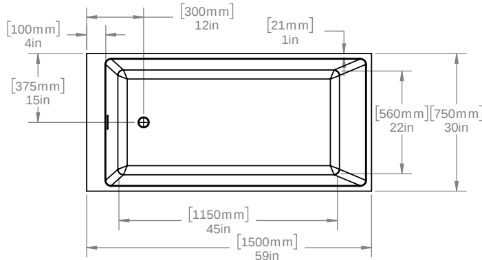
TOP VIEW VUE DE DESSUS
