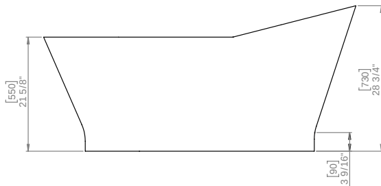
FRONT VIEW VUE DE FACE
