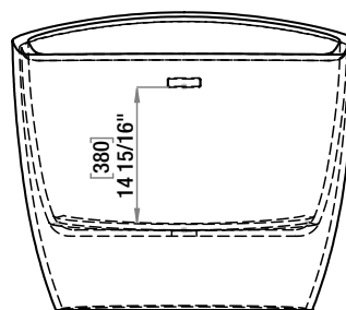
SIDE VIEW VUE DE CÔTÉ
