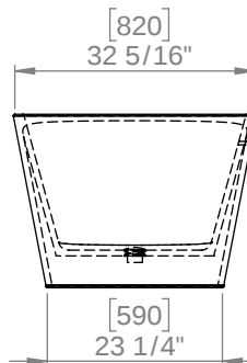
SIDE VIEW VUE DE CÔTÉ
