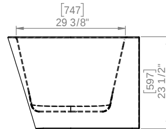
SIDE VIEW VUE DE CÔTÉ
