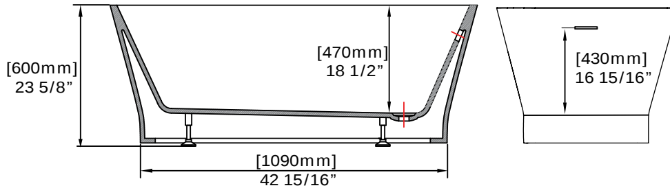
FRONT VIEW VUE DE FACE
