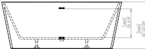
FRONT VIEW VUE DE FACE
