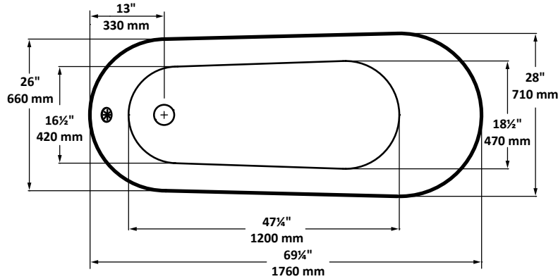
TOP VIEW VUE DE DESSUS
