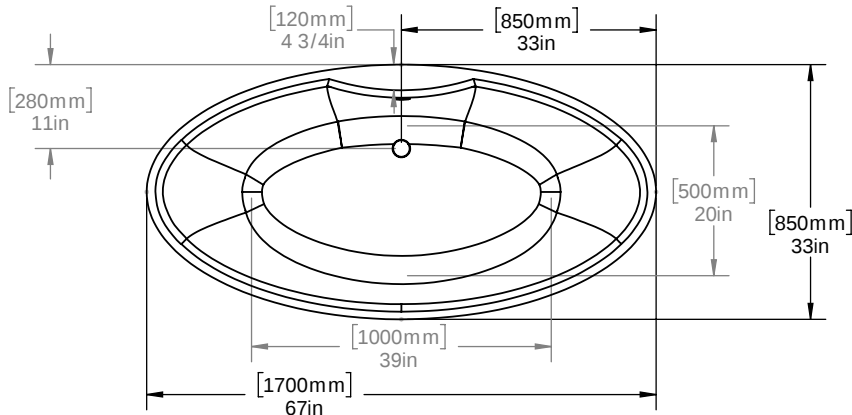
TOP VIEW VUE DE DESSUS
