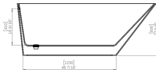
FRONT VIEW VUE DE FACE
