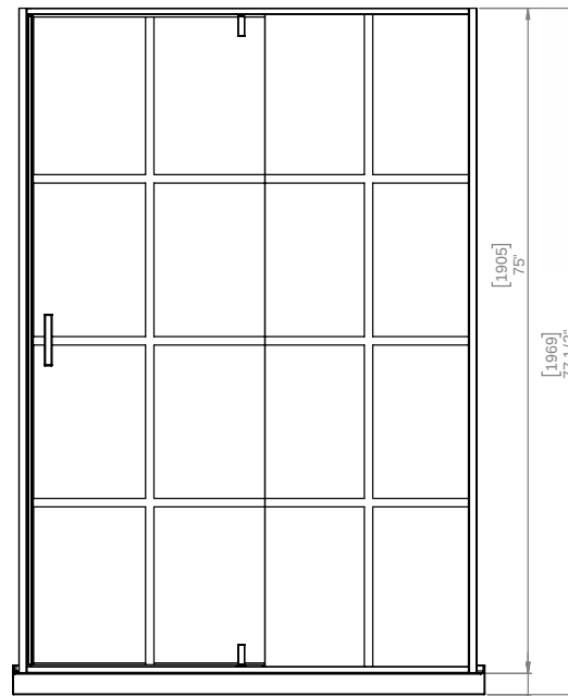
FRONT VIEW VUE DE FACE
