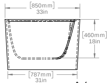
SIDE VIEW VUE DE CÔTÉ
