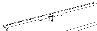
Barrette d'écoulement (percée) avec entretoises (S65-476A)
