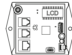
Caja de control maestro (S39-845) Tornillo n.º 10 x 3/8" (2x) (P18-054)
