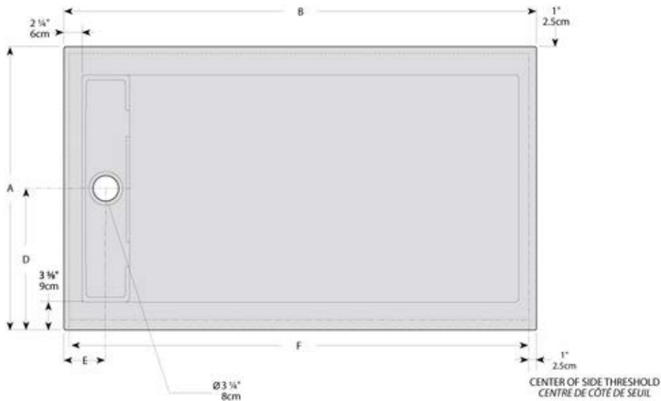
FRONT VIEW VUE DE PROFIL
