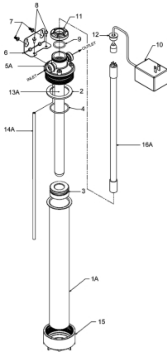
UV Addon 3 GPM
