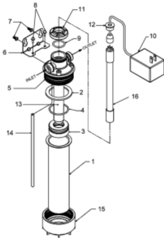
UV Addon 1 GPM
