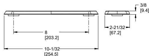
Optional Deckplate
